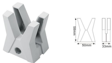
PFJ-21 卡口铝合金屏风夹 Bayonet aluminum screen clip
