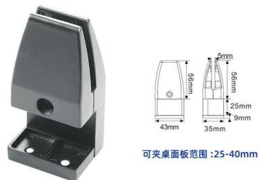
PFJ-22 巴黎夹 Paris clip
